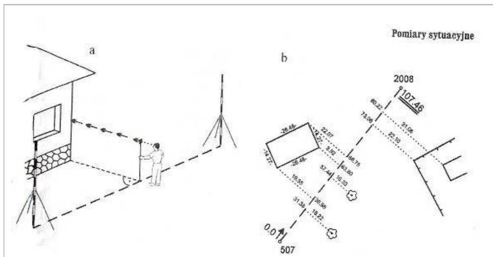
Rysunek 3.6 Pomiar szczegółów metoda domiarów prostokątnych i sposób zapisu na szkicu
