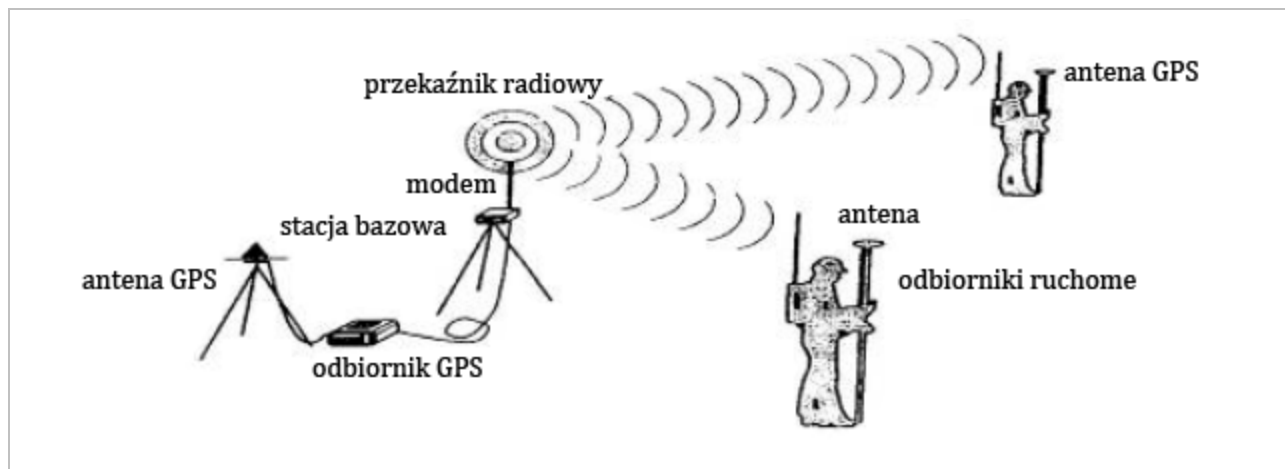
Rysunek 3.9 Zasada pomiarów terenowych GPS
