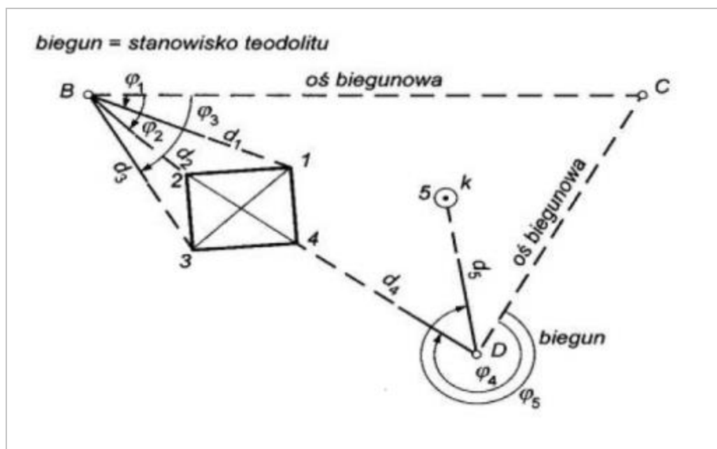
Rysunek 3.5 Pomiar sytuacji metodą biegunową
