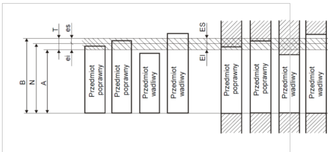
Rysunek 3.11 Wymiary: nominalny, graficzny, tolerancji wymiaru i odchyłki
